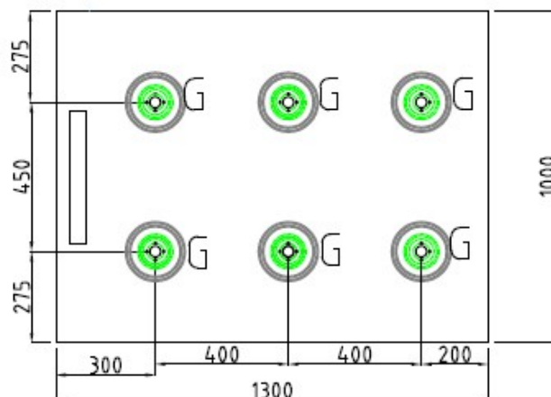
10PCFLG6PA/12
